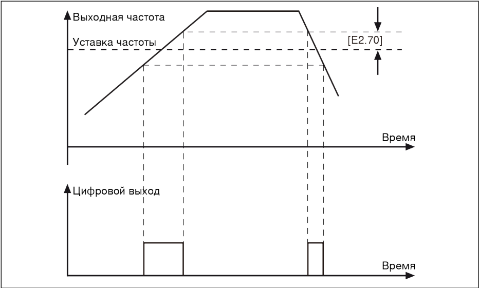
Рис. 12-34: Достижение частоты
