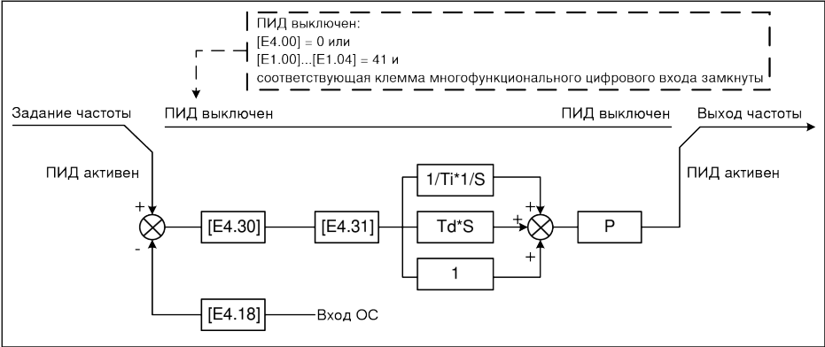
Рис. 12-40: Отключение ПИД с помощью цифрового входа
