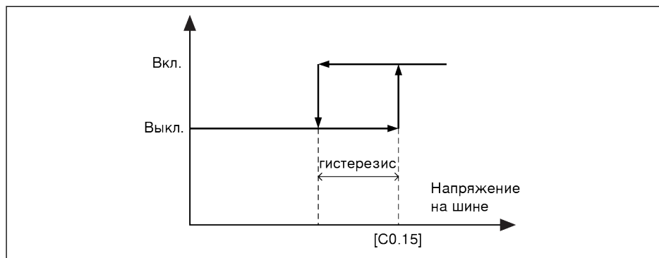
Рис. 12-25: Гистерезис
