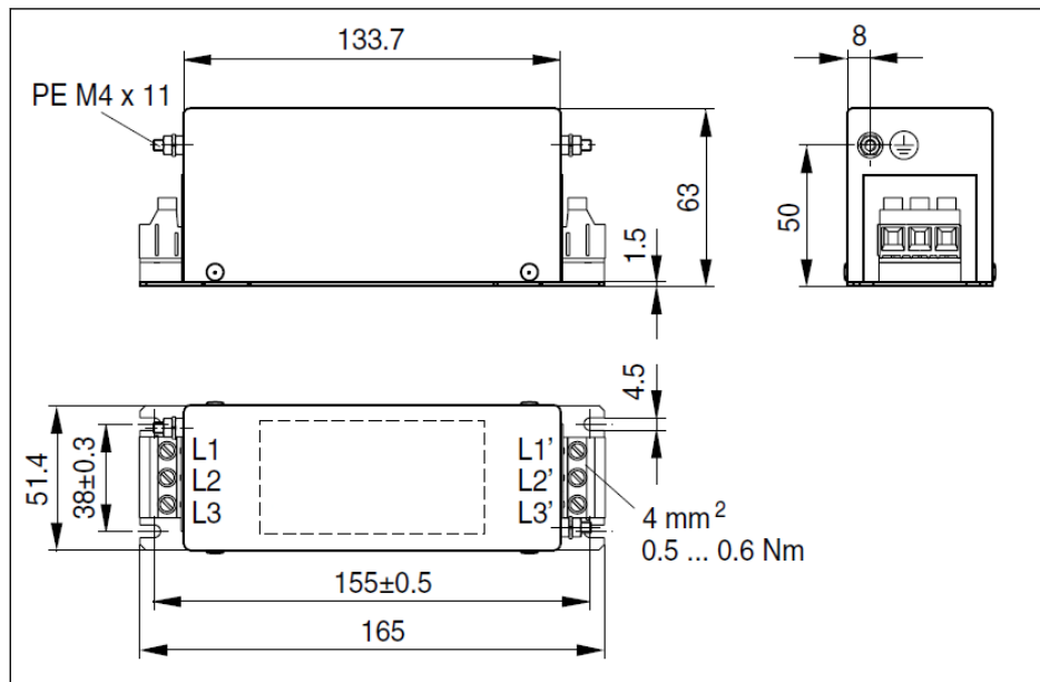
Рис. 15-4: E0008-A-480
