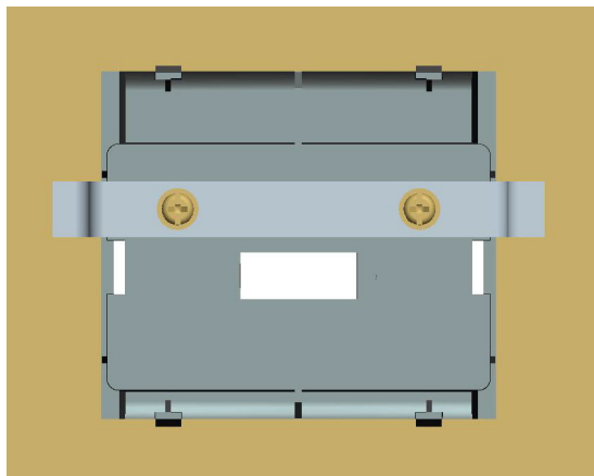
Рис. 15-13: Зафиксируйте монтажную плату (вид сзади)
