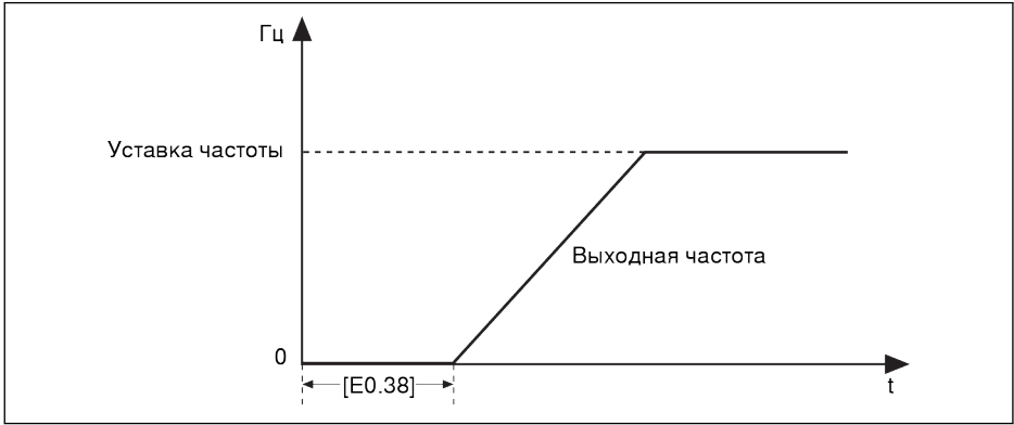
Рис. 12-20: Торможение пост. током перед запуском
