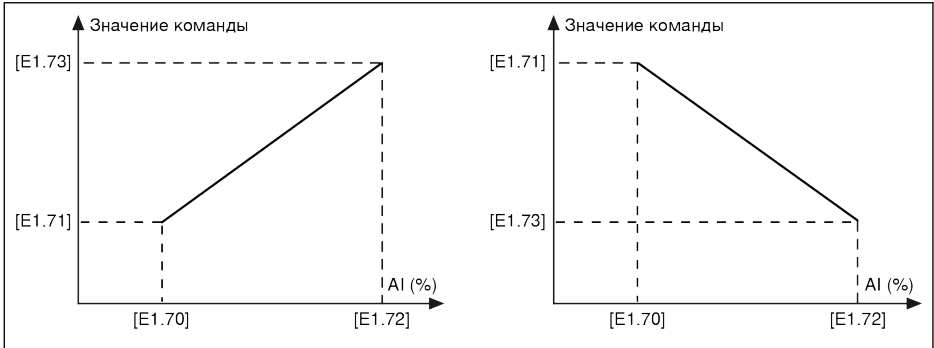
Рис. 12-1: Кривая 1
