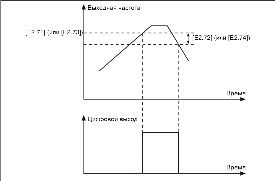
Рис. 12-35: Обнаружение уровня частоты
