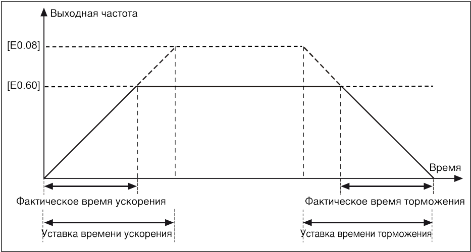
Рис. 12-27: Время ускорения/торможения в толчковом режиме
