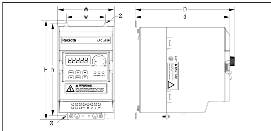
Рис. 7-2: Размерный чертеж VFC x610 0K40...4K00
