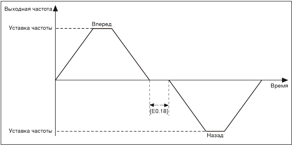
Рис. 12-18: Время задержки смены направления
