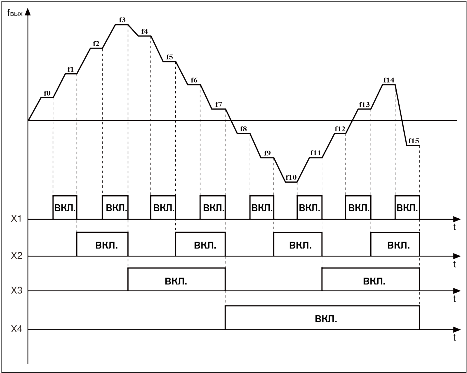
Рис. 12-11: Переход в фазу многоскоростного режима
