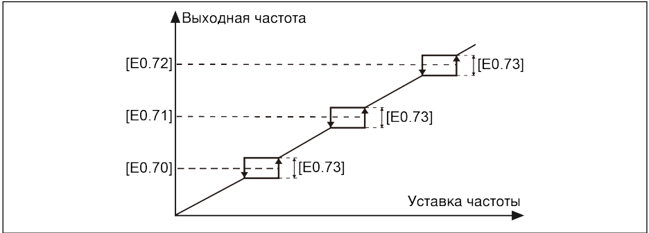
Рис. 12-26: Частота пропуска
