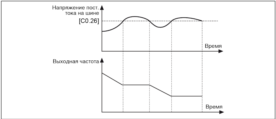
Рис. 12-43: Предотвращение скачков напряжения при замедлении
