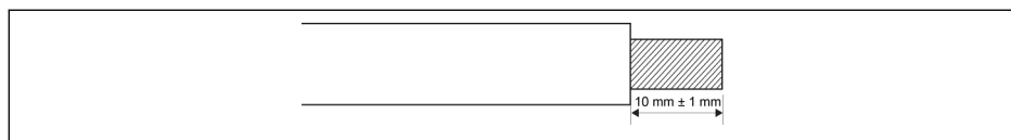
Рис. 8-2: Длина зачистки изоляции кабелей
