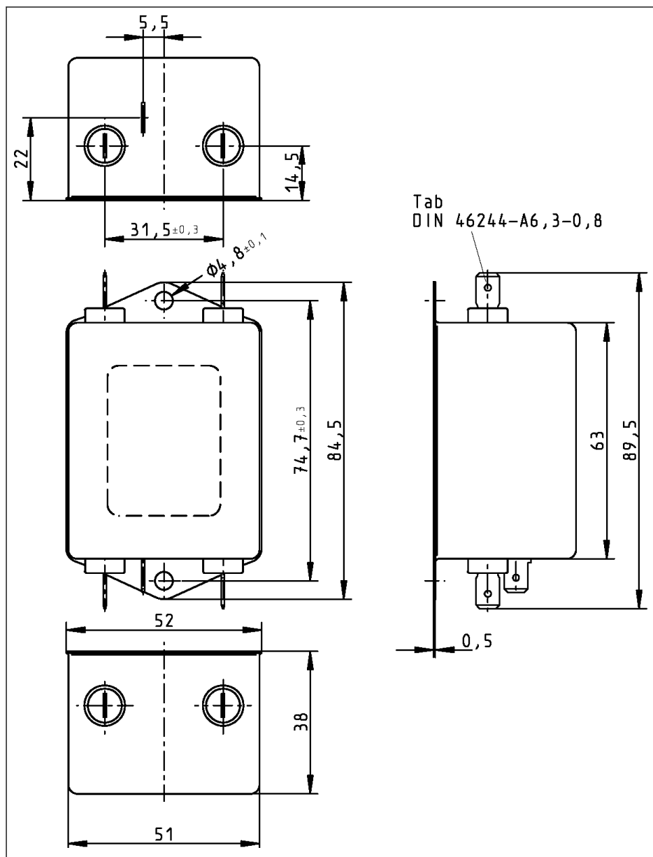
Рис. 15-1: E0006-A-240
